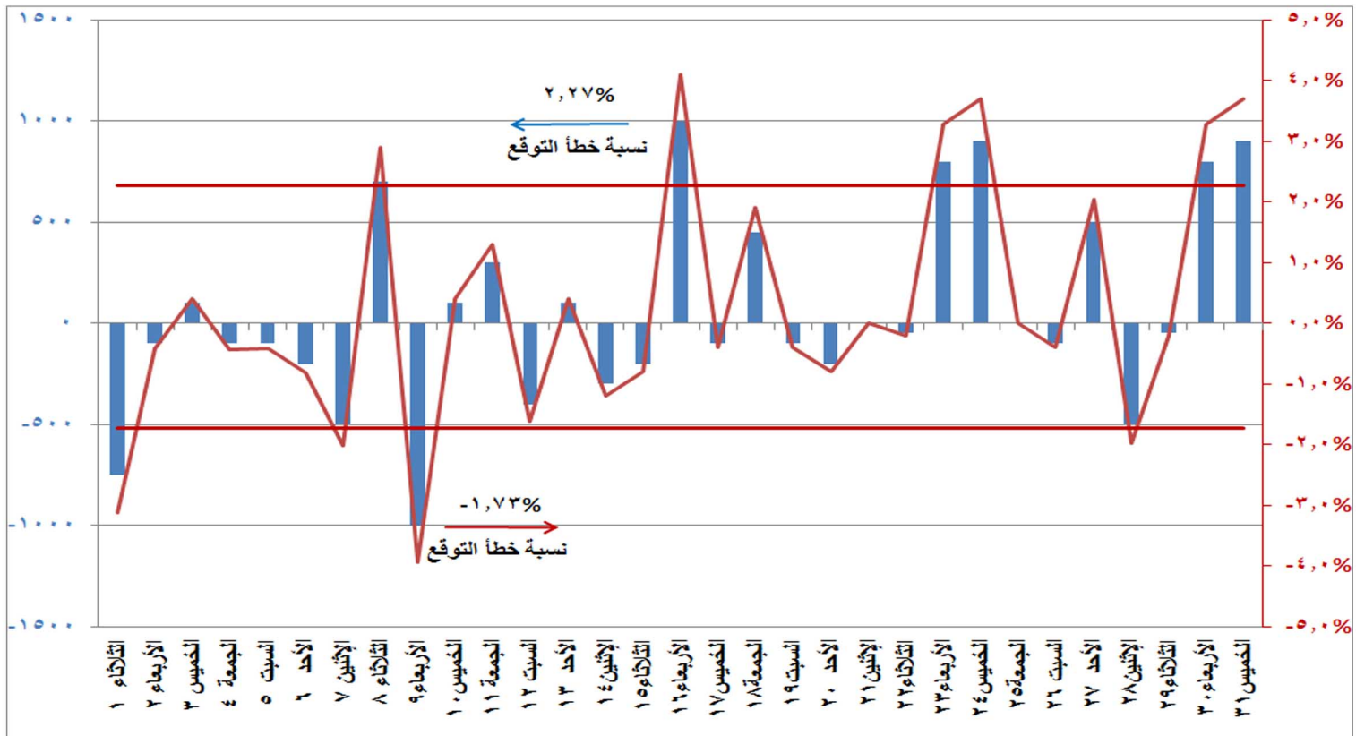
شكل (١٠) الفرق بين الحمل الأقصى المتوقع والمسجل فعلياً ونسبة الفرق إلى الحمل المسجل فعلياً خلال شهر يناير ٢٠١٩
