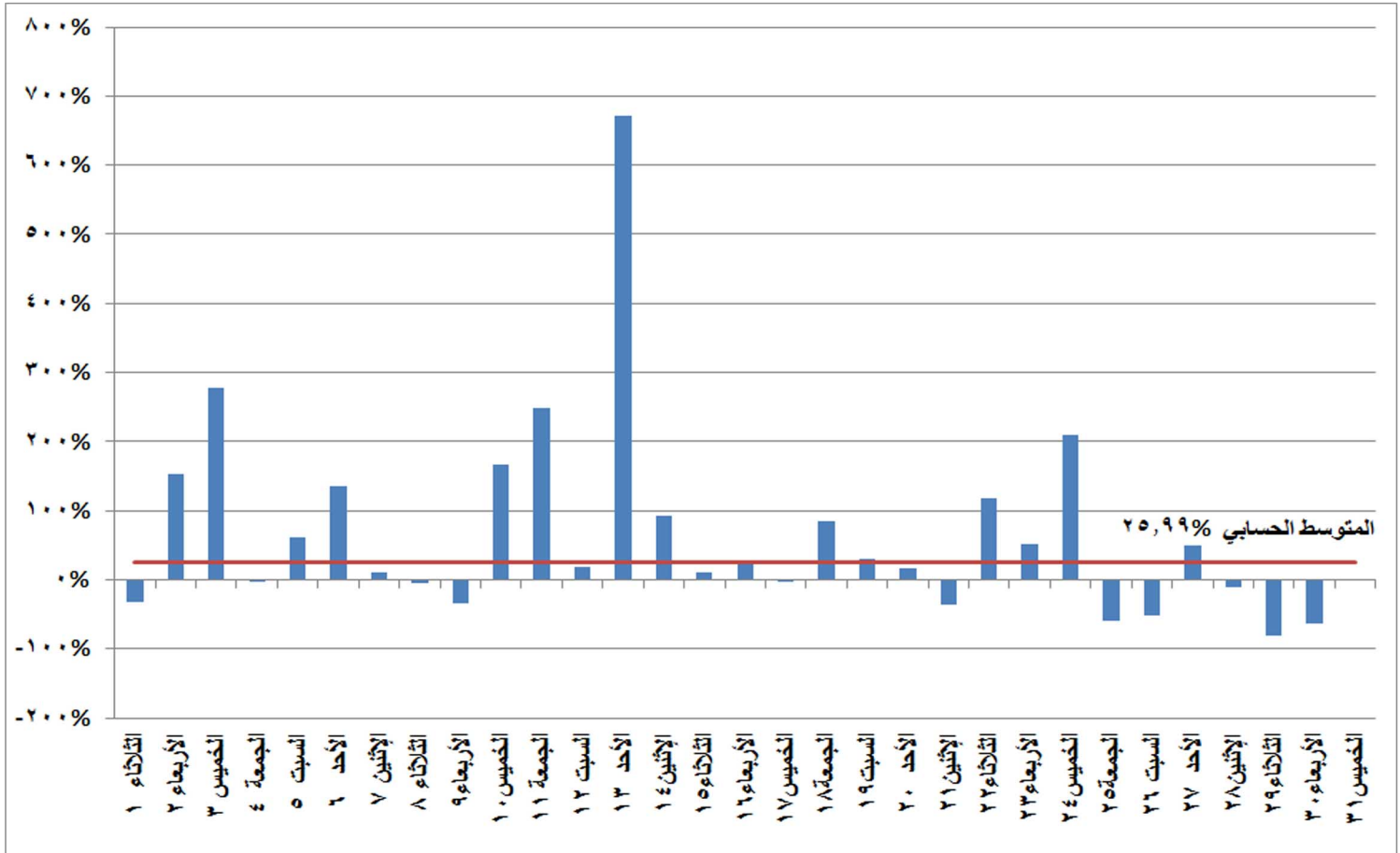
شكل (٢٦) نسب التغير في استخدام الرياح والشمس في إنتاج الطاقة الكهربائية خلال شهر يناير ٢٠١٩ مقارنة بالشهر المماثل من العام السابق
