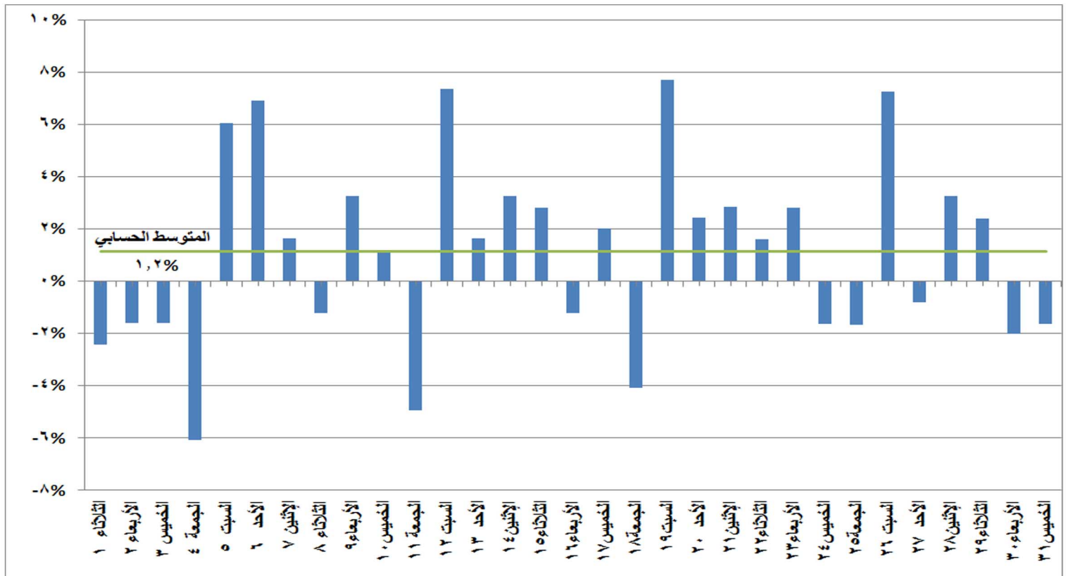
شكل (٩) النسب المئوية للتغير في الحمل الاقصى خلال شهر يناير ٢٠١٩ مقارنة باليوم المماثل من العام الماضي
