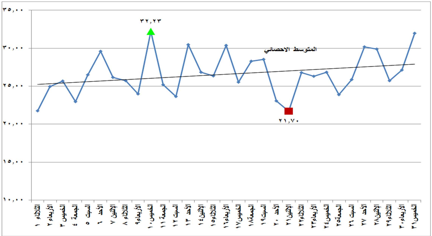
شكل (٢١) الطاقة الكهربائية المنتجة من المصادر غير الحرارية خلال شهر يناير ٢٠١٩
