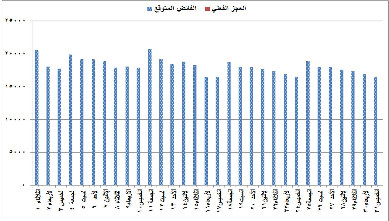
شكل (٧) الفائض والعجز المتوقع للقدرات خلال شهر يناير ٢٠١٩
