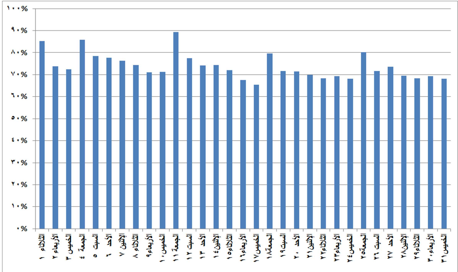
شكل (٢٨) نسب الفائض للحمل الاقصى المسجل يوميا خلال شهر يناير ٢٠١٩
