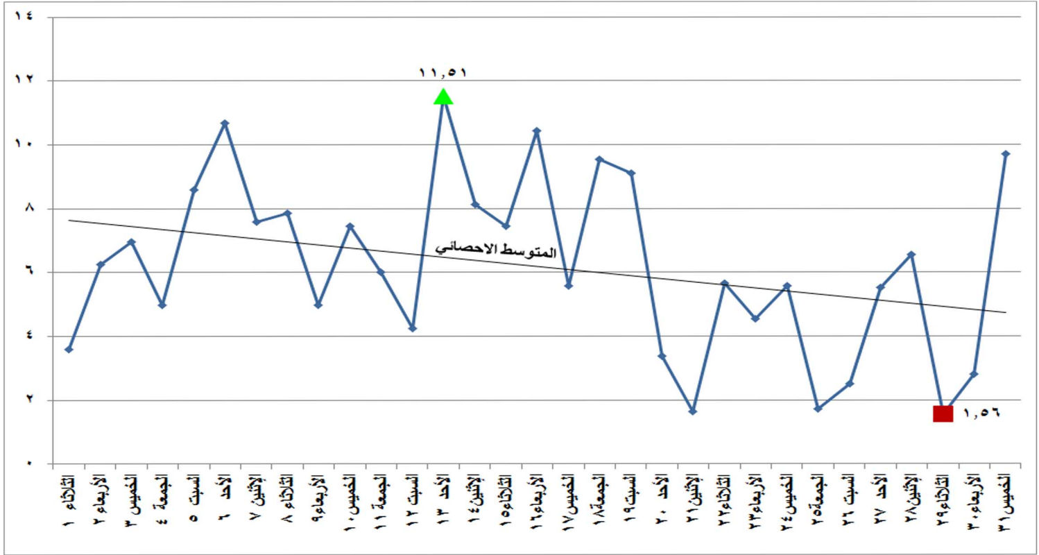
شكل (٢٥) الطاقة الكهربائية المنتجة من الرياح والشمس خلال شهر يناير ٢٠١٩
