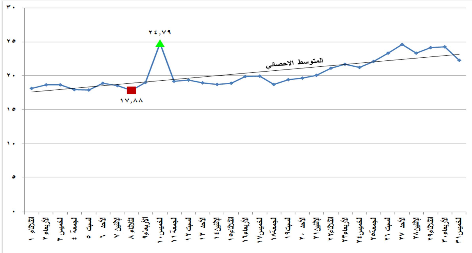
شكل (٢٣) الطاقة الكهربائية المنتجة من المصادر المائبة خلال شهر يناير ٢٠١٩
