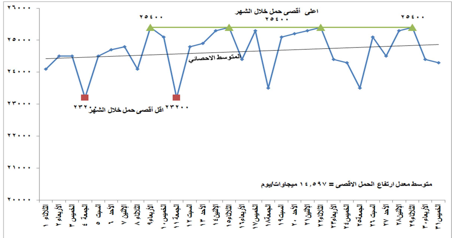
شكل (١) تطور الحمل الاقصى اليومي خلال شهر يناير ٢٠١٩
