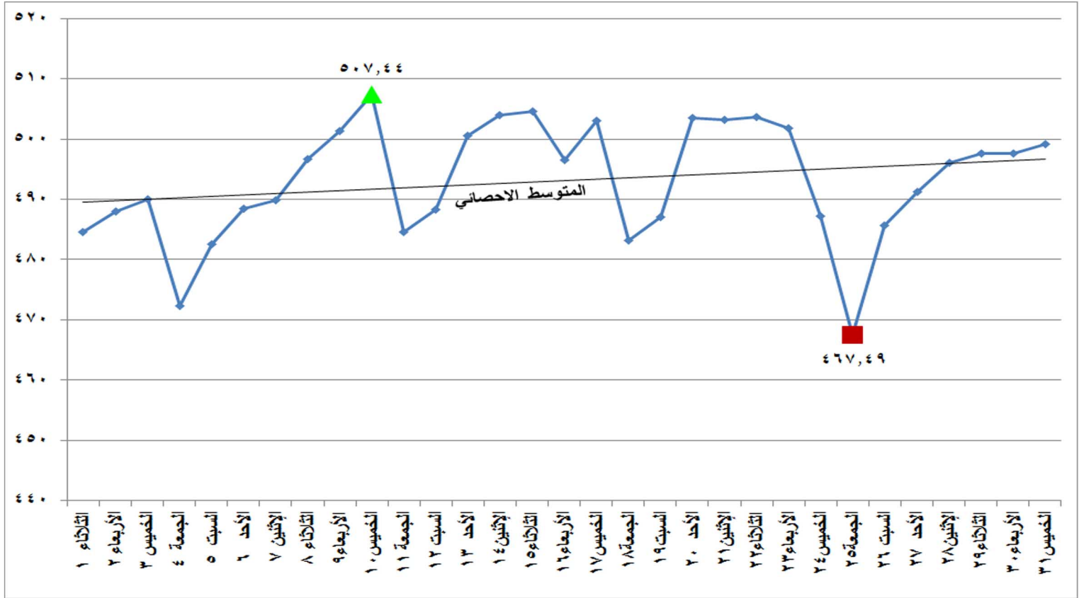
شكل (١٥) إجمالي الطاقة الكهربائية المنتجة من كل المصادر الأولية خلال شهر يناير ٢٠١٩
