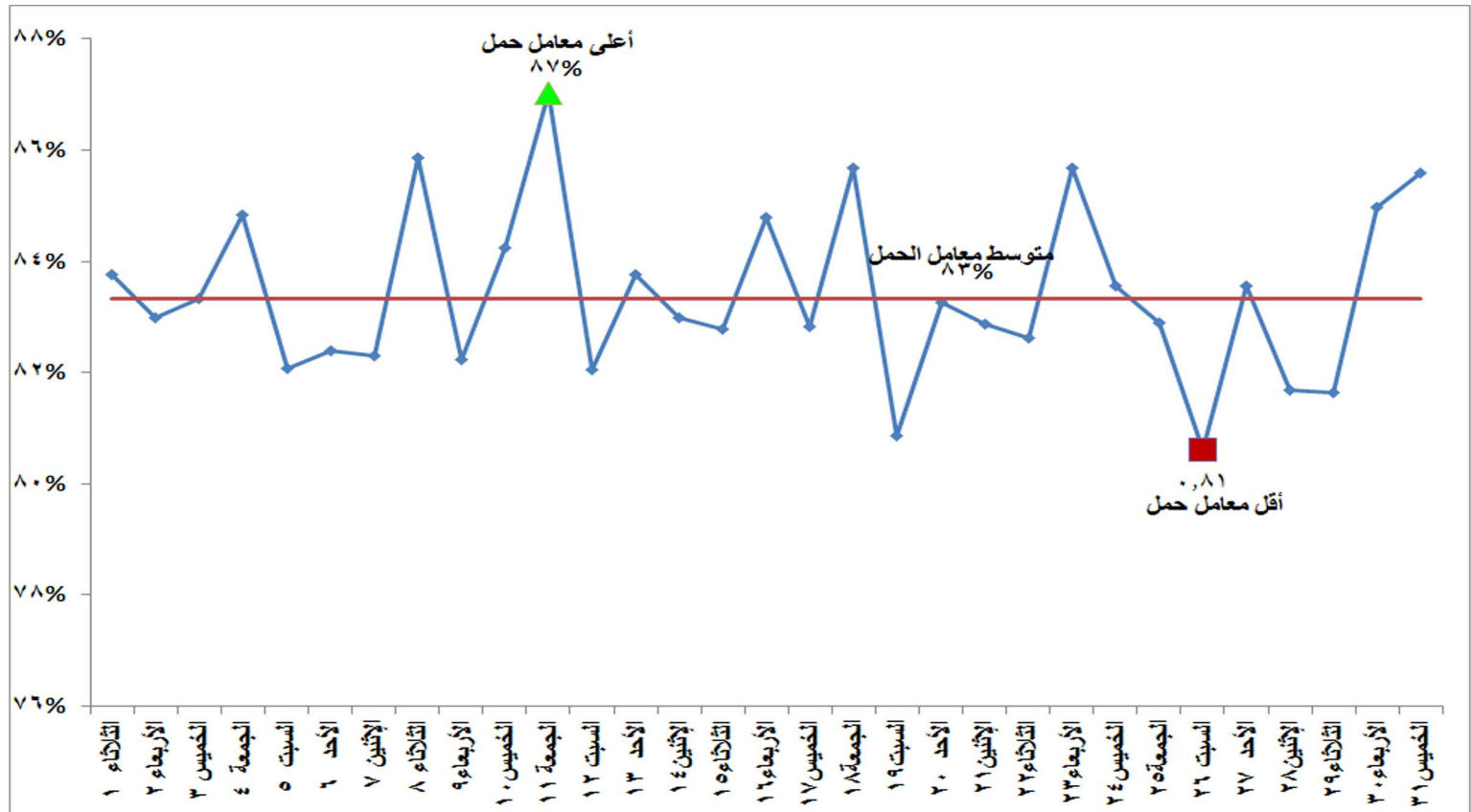
شكل (١٢) إجمالي معامل الحمل لوحدات الانتاج خلال شهر يناير ٢٠١٩
