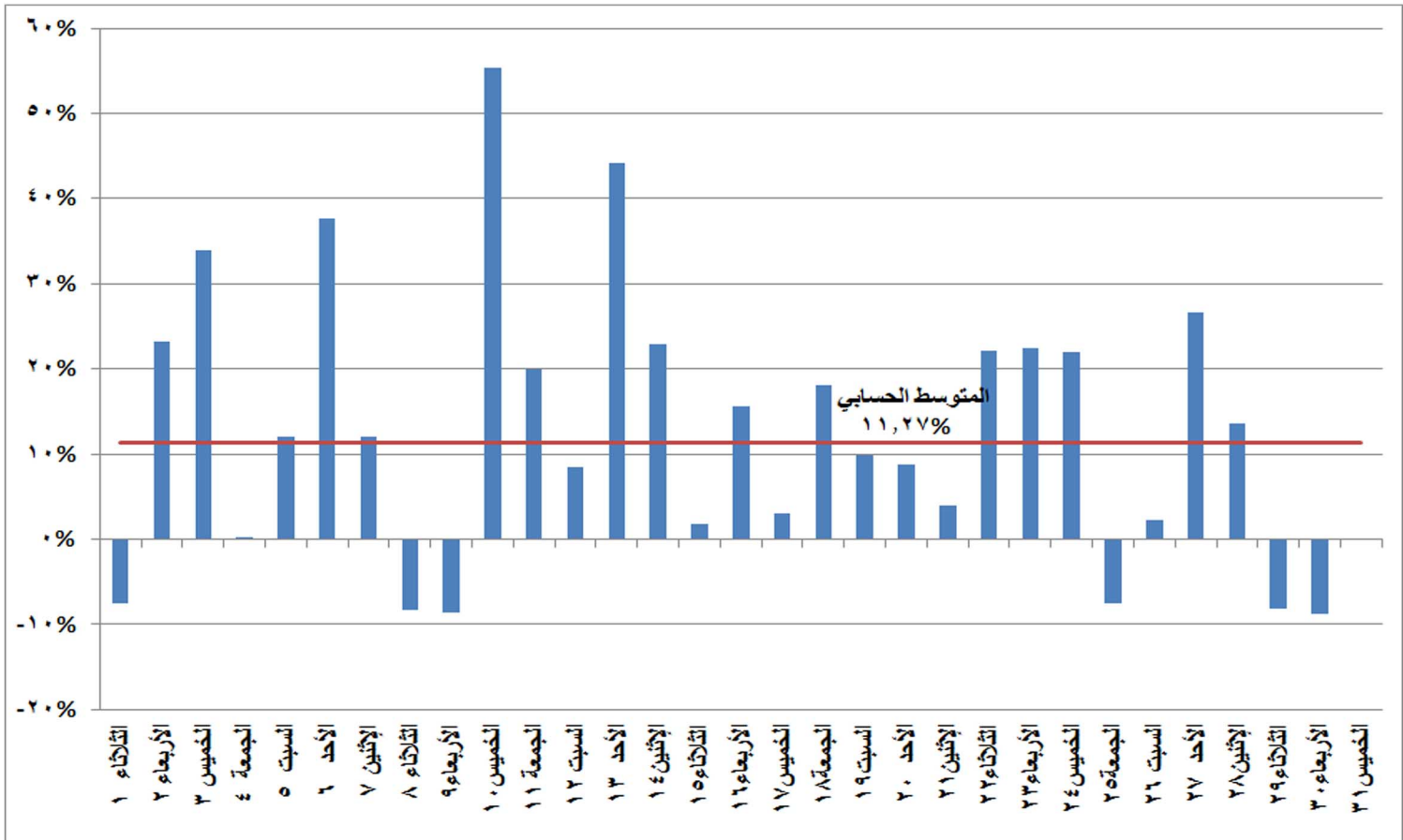
شكل (٢٢) نسب التغير في استخدام المصادر غير الحرارية في إنتاج الطاقة الكهربائية خلال شهر يناير ٢٠١٩ مقارنة بالشهر المماثل من العام السابق
