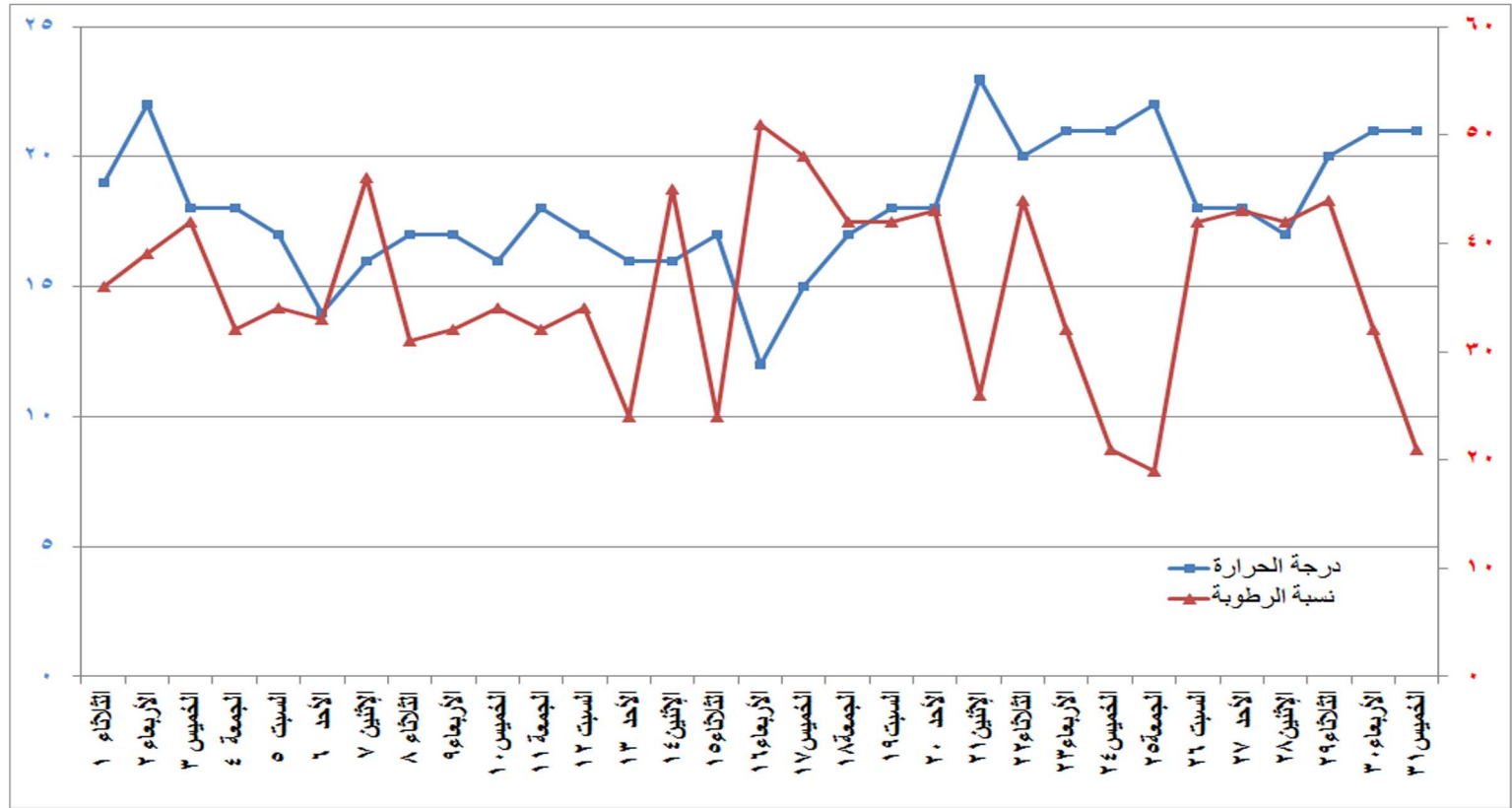
شكل (١١) التغيير في درجة الحرارة والرطوبة النسبية خلال شهر يناير ٢٠١٩
