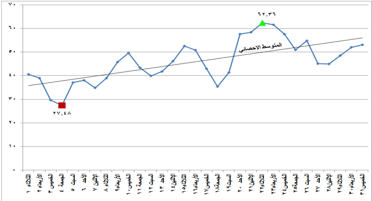
شكل (١٩) الطاقة الكهربائية المنتجة من المازوت خلال شهر يناير ٢٠١٩
