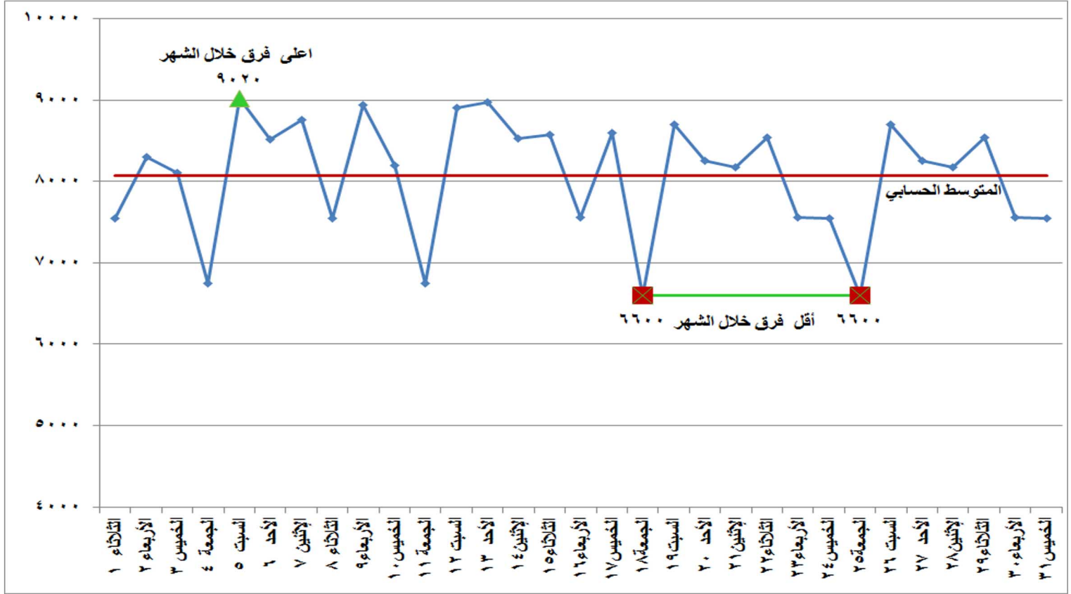
شكل (٣) الفرق بين أقصى وأدنى حمل خلال شهر يناير ٢٠١٩
