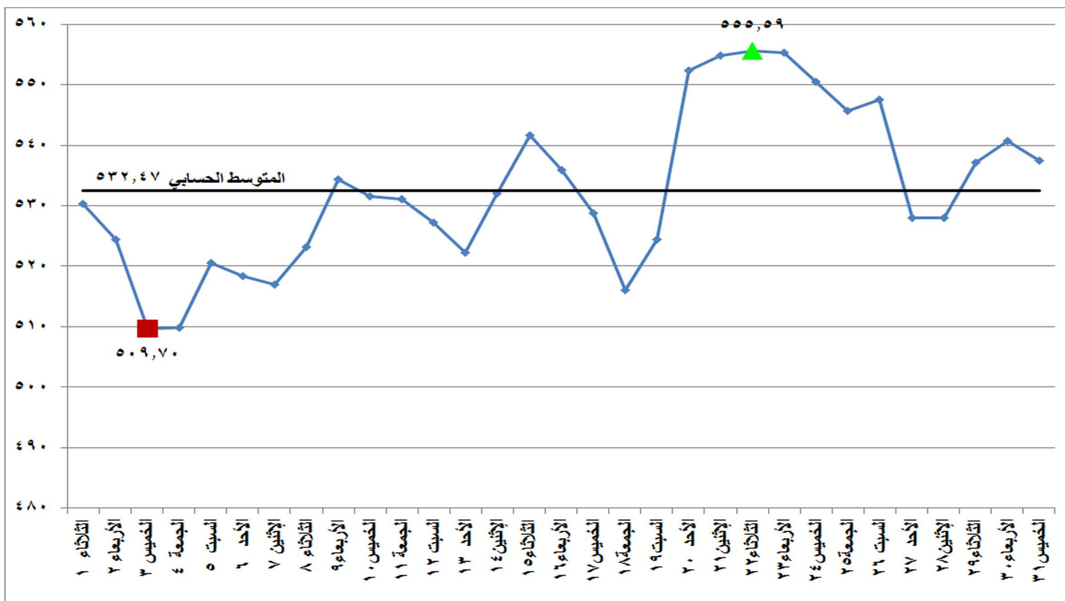
شكل (١٤) معامل انبعاثات غاز ثاني اكسيد الكربون المكافئ على مدى شهر يناير ٢٠١٩
