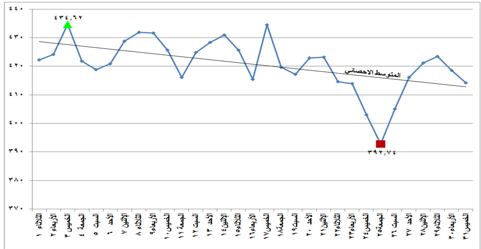
شكل (١٧) الطاقة الكهربائية المنتجة من الغاز الطبيعي خلال شهر يناير ٢٠١٩
