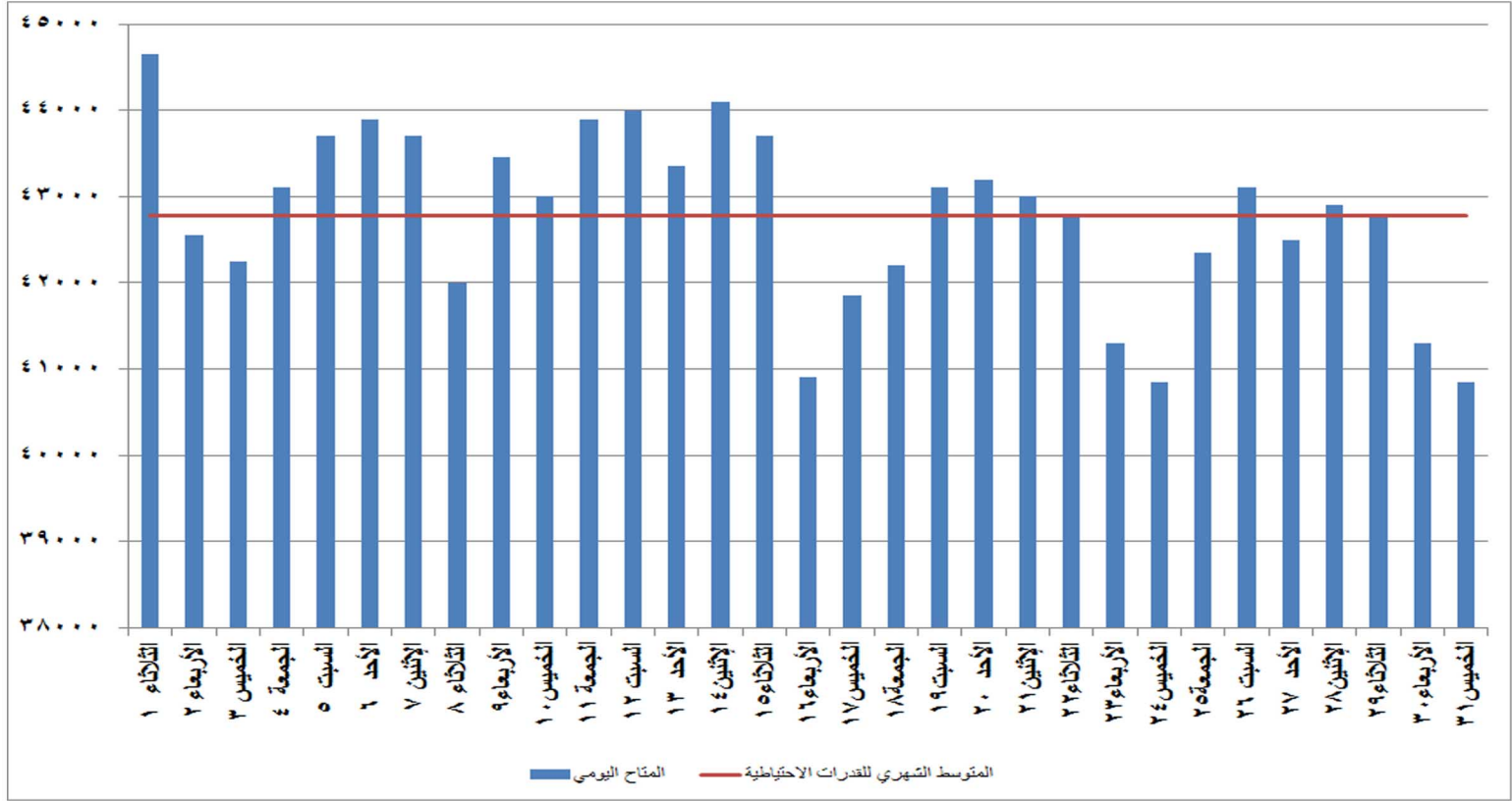
شكل (٢٧) القدرات المتاحة يوميا والمتوسط الشهري للقدرة الاحتياطية خلال شهر يناير ٢٠١٩
