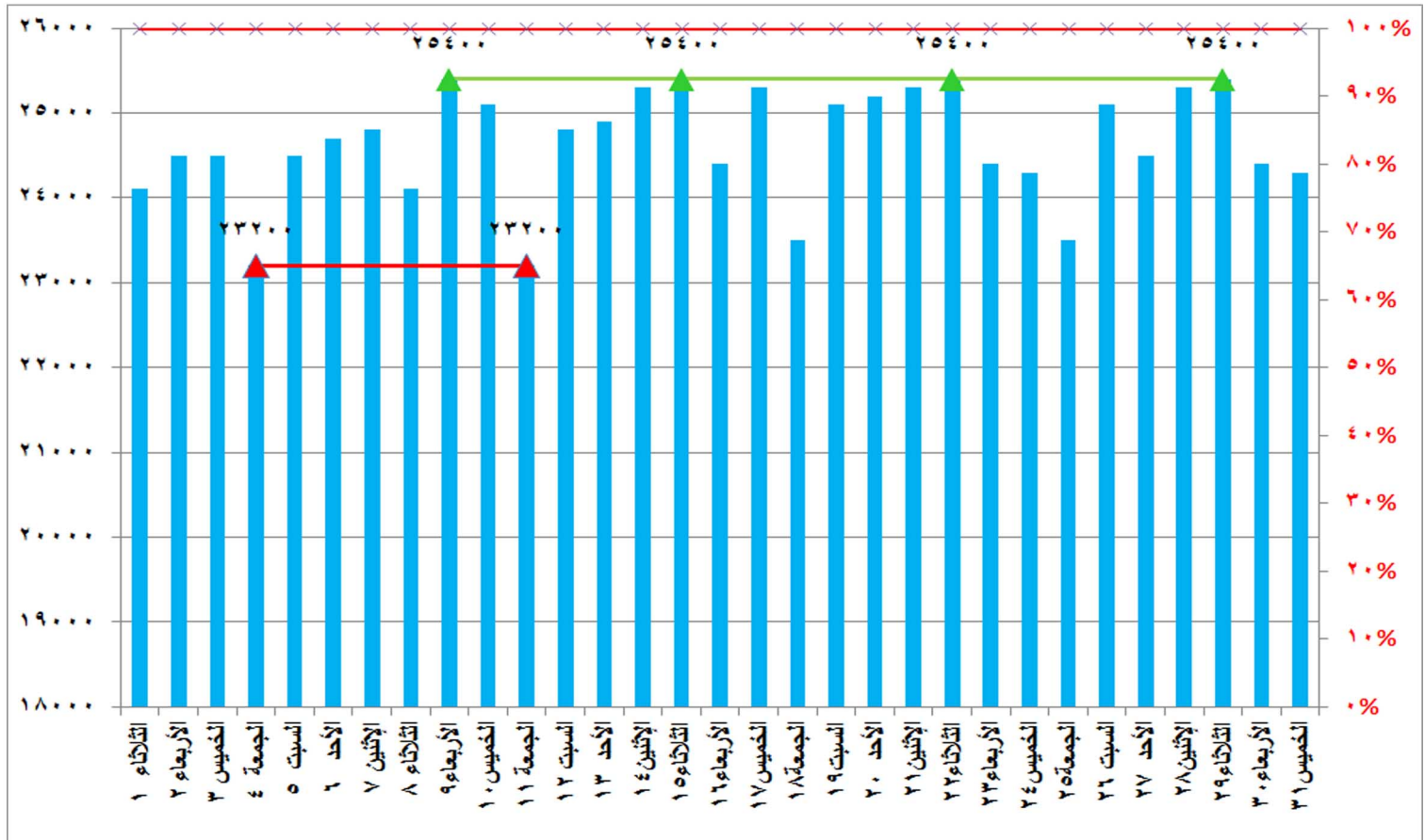
شكل (٥) قدرات الانتاج المتاحة ونسبتها للحمل الأقصى خلال شهر يناير ٢٠١٩
